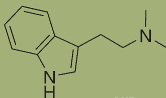
DMT
